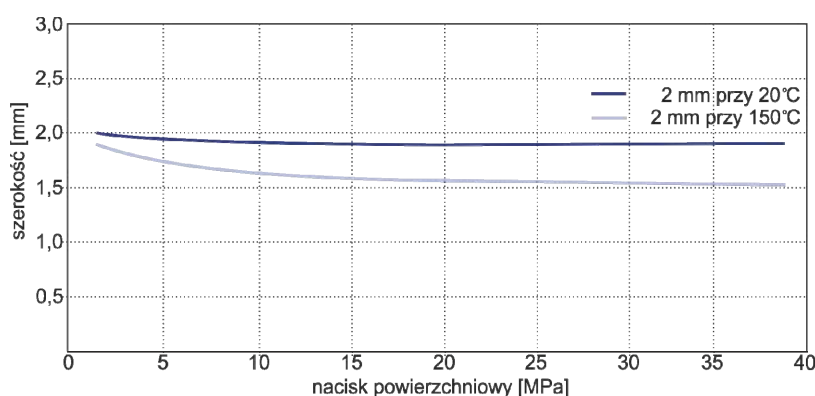
Zmiana grubości uszczelki w zależności od nacisku powierzchniowego przy temp. 20°C i przy 150°C
