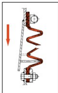
Rys 11. Profil E-1 – kompensator mieszkowy mocowany na opaski
