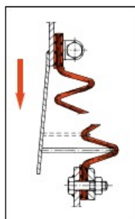
Rys 12. Profil E-15 – Kompensator redukcyjny mieszkowy mocowany na opaski
