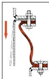
Rys 15. Profil E-3 – Kompensator mieszkowy – wykonanie kołnierzone z wewnętrznymi i zewnętrznymi pierścieniami stalowymi
