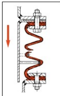
Rys 15. Profil E-3 – Kompensator mieszkowy – wykonanie kołnierzone z wewnętrznymi i zewnętrznymi pierścieniami stalowymi
